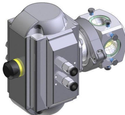
Drie- weg rotatie klep DN 15
